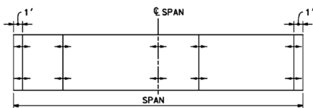
ELEVATION (3)
